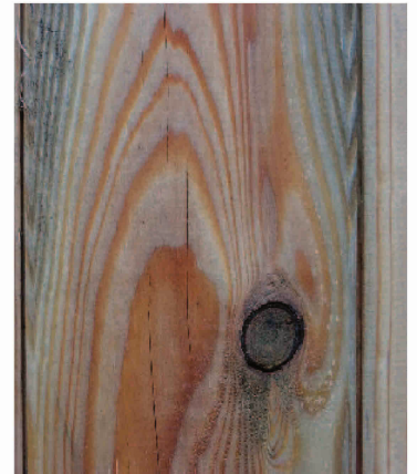
Abb. 5: Detailansicht, das Splintholz wird intensiver durch Bläue- und Schimmelpilze bewachsen als das dunklere Kernholz.
