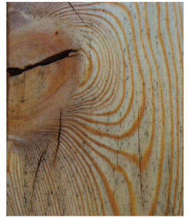
Abb. 4: Detailansicht, Trocknungsrisse im Bereich eines Astes, zudem beginnender Bewuchs durch Bläue- und Schimmelpilze.
