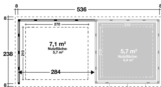
Grundriss: Beispiel Eleganto 2424 inkl. Loungeanbau links
