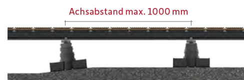
VARIO FIX mit Konstruktionsbalken 80 x 60 mm
