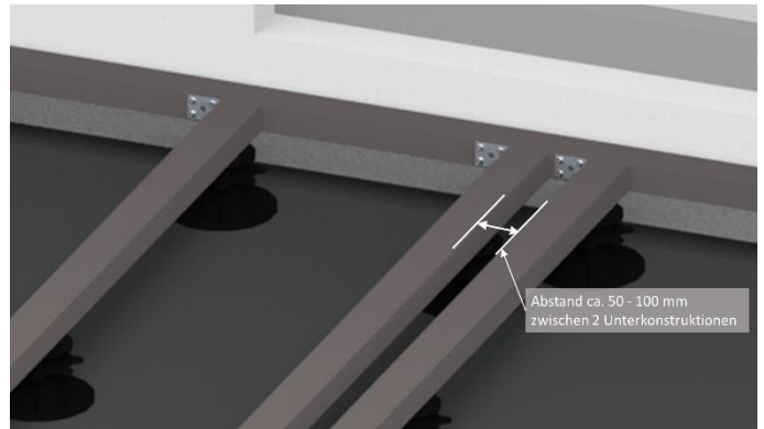
Bild 9. An Längsstößen der Terrassendielen müssen 2 Unterkonstruktionen mit einem Abstand von ca. 50 – 100 mm eingebaut werden.
