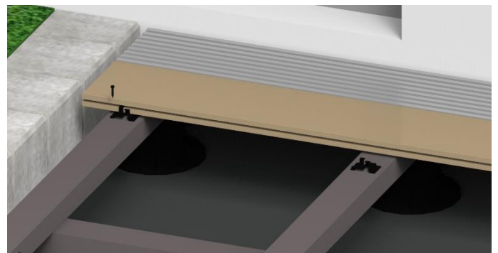
Bild 22. Die WPC-Diele wird mit dem notwendigen Abstand ausgerichtet und die Befestigungsclipse unter die Diele geschoben.
