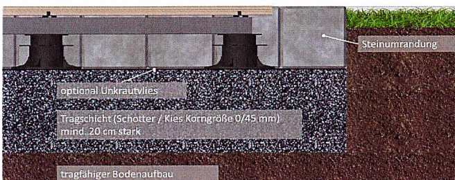
Bild 1. Die Tragschicht sollte je nach Ausführung ca. 15- 20 cm stark sein.
