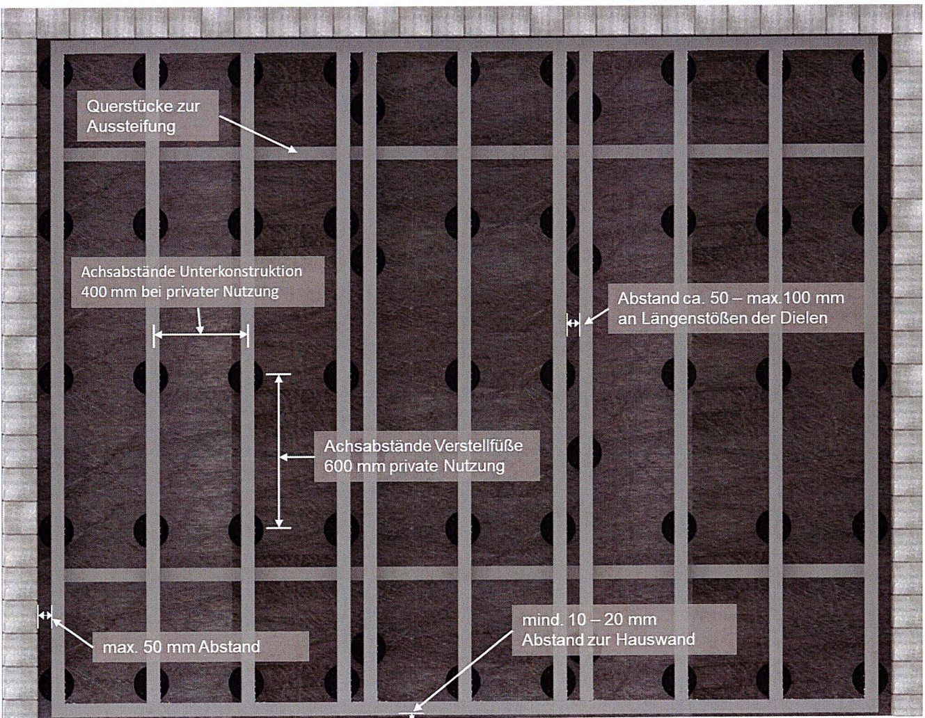
Bild 14. Schematische Darstellung für eine ausgesteifte Rahmenkonstruktion mit Verstellfüßen auf einer Tragschicht mit Schotter Korngröße 0-45 und einem zusätzlichen wasserdurchlässigen Unkrautvlies. Die maximale Belastung darf 2 kN/m 2 nicht überschreiten. Bei höheren Lasten bzw. unter Blumenkästen oder Sonnenschirmständern, müssen weitere Unterkonstruktionen und Verstellfüße eingeplant werden.
