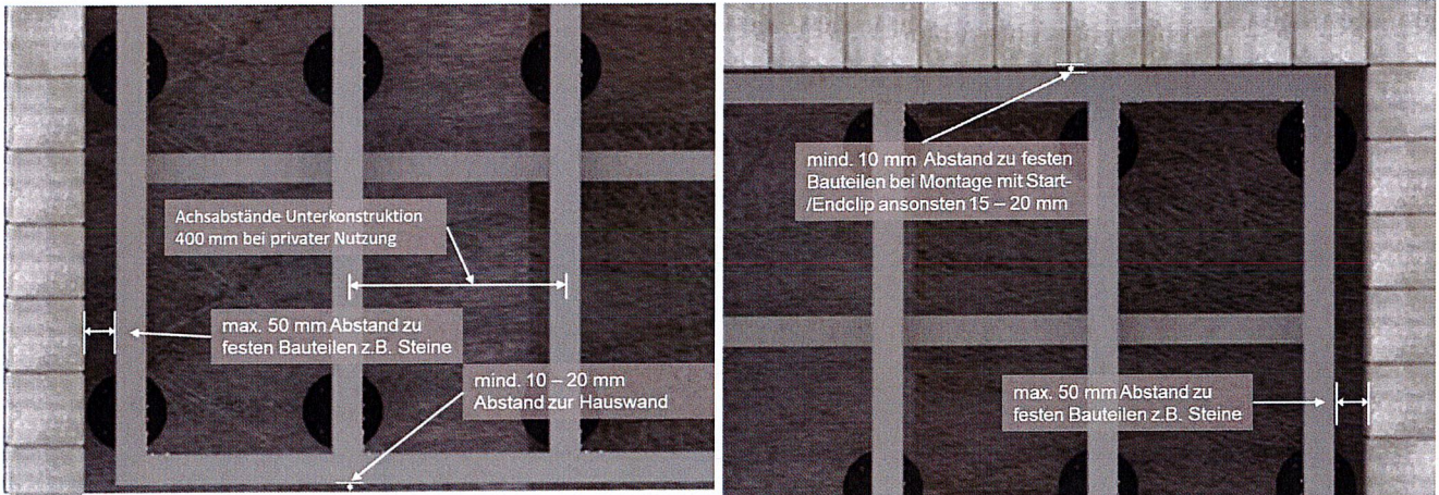
Bild 12 + 13. Durch die Größe der Bodenplatte unser Verstellfüße von ca. 160 mm wird der Abstand der Unterkonstruktion zu der Steinumrandung definiert und sollte max. 50 mm betragen. Wenn möglich sollten die Verstellfüße an die Außenkante der rechten und linken Unterkonstruktion geschraubt werden. Zur Hauswand und festen Bauteilen z.B. Steinumrandung, muss der Abstand der vorderen und hinteren Unterkonstruktion ca. 10 – 20 mm betragen. Bei der Verwendung der Anfangsclipse für die erste und letzte WPC-Diele, sollte nur 10 mm Abstand eingeplant werden da die WPC-Diele ca. 10 – 13 mm zurückspringt.
