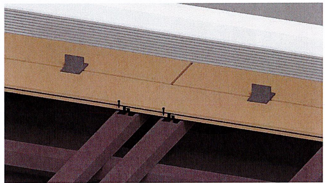
Bild 17. Mit Abstandshaltern kann einfach eine ca. 1 mm größere Fuge sichergestellt werden als die Befestigungssysteme vorgeben.
