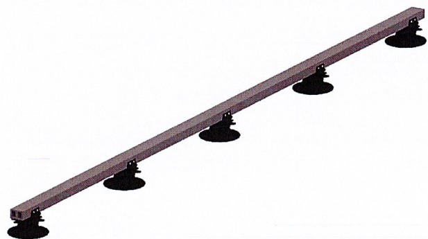
Bild 5. Die Verstellfüße müssen mit einem maximalen Achsabstand von 600 mm an die WPC-Unterkonstruktionen geschraubt werden.
