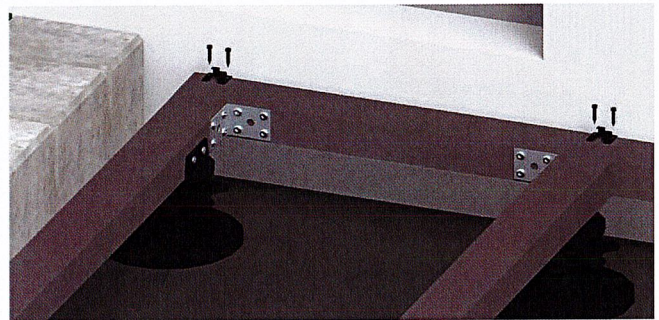
Bild 20. Wenn kein Entwässerungsrost erforderlich ist, wird der Anfangsclip bündig mit der hinteren Kante der Unterkonstruktion montiert.
