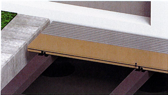
Bild 23. Mit je 1 Edelstahlschraube 4,2 x 22 mm wird der Befestigungsclip auf der Unterkonstruktion verschraubt. Bitte beachten Sie das die Verschraubung mit dem richtigen Drehmoment erfolgt (ca. 3,6 Nm).
