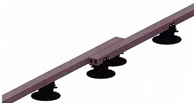
Bild 4. Bei langen Längen müssen die WPC-Unterkonstruktionen versetzt angeordnet werden.
