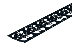
TRAGPROFIL FLACH Material: Normalstahl geschwärzt Länge 960 mm
